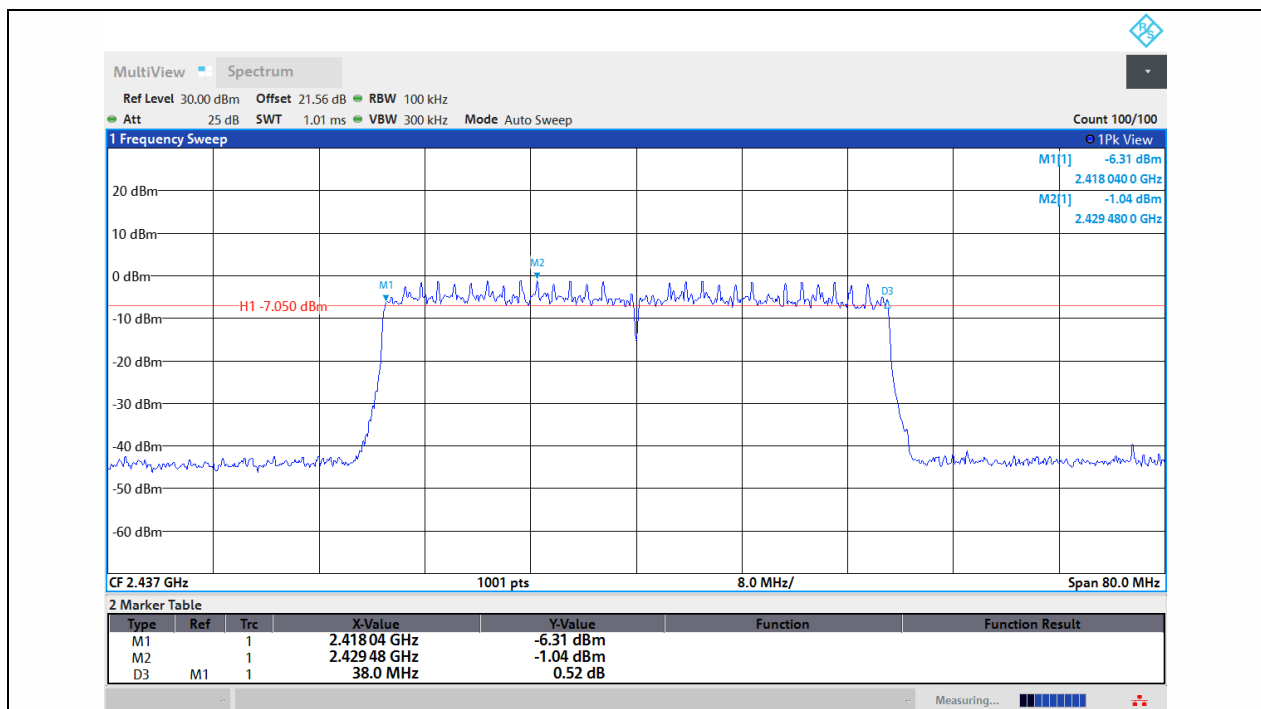
11AX40MIMO-Ant1-2437-PASS
