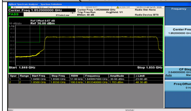
Band2-5MHz-QPSK-18625-25RB#0-PASS
