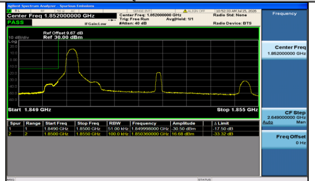
Band2-5MHz-16QAM-18625-1RB#0-PASS
