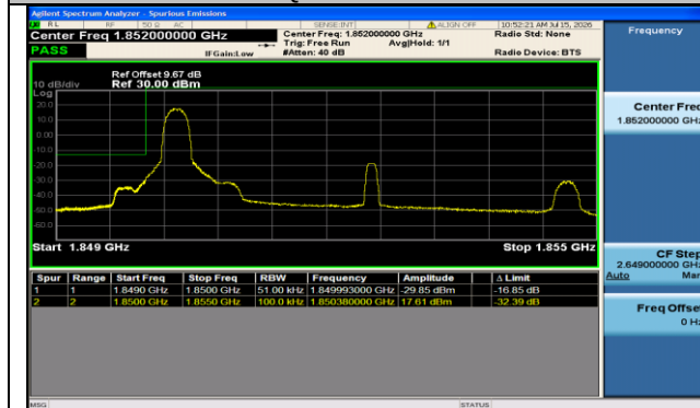
Band2-5MHz-QPSK-18625-1RB#0-PASS
