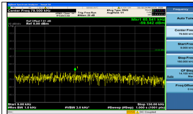
Band5-3MHz-QPSK-20635-15RB#0-0.009~0.15-PASS
