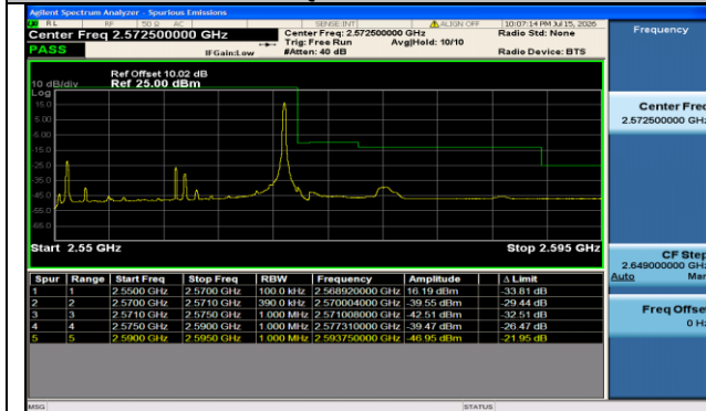
Band7-20MHz-QPSK-21350-1RB#99-PASS
