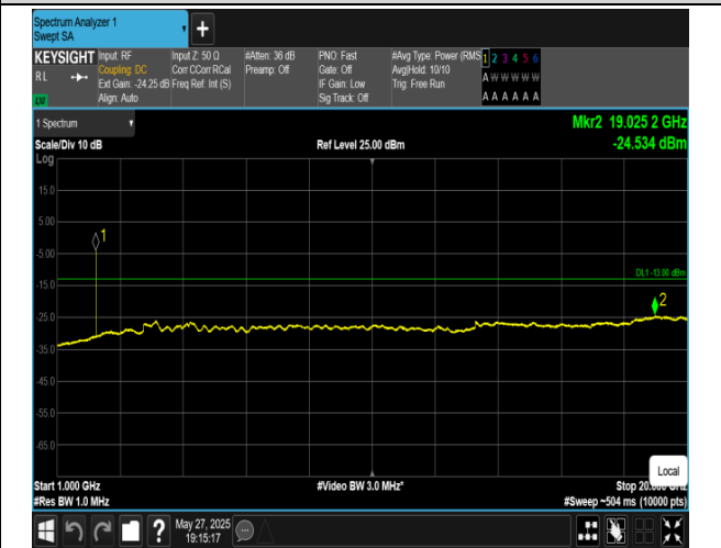
Band66-5MHz-QPSK-67111-E-TM1.1-1000~20000
