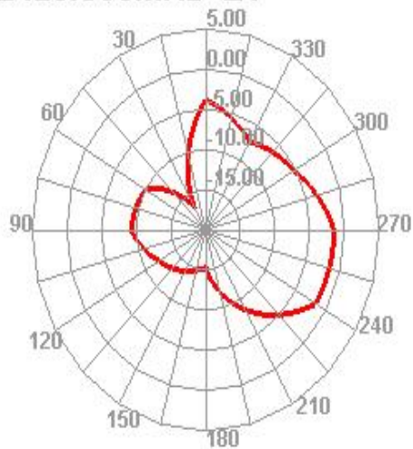
2420.000MHz E1
