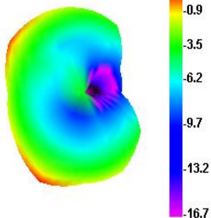
2410.000MHz E1
