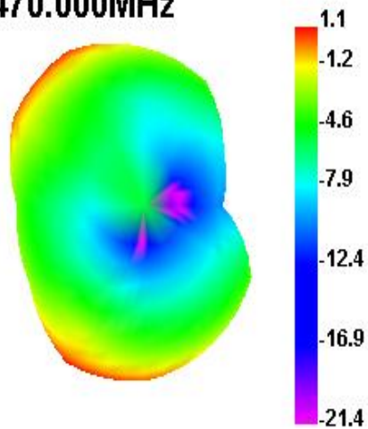
2470.000MHz
