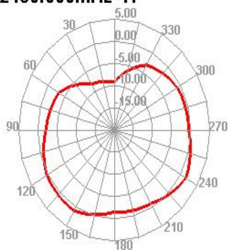
2430.000MHz H
