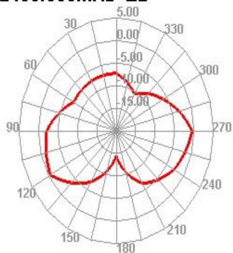
2430.000MHz E2
