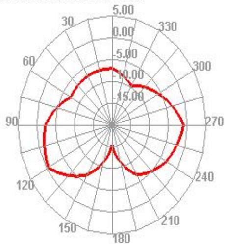
2420.000MHz E2
