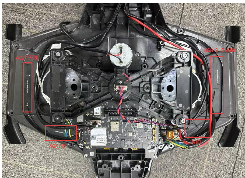
Antenna
