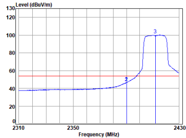
11g_TX_CH_01_Horizontal-Avg
