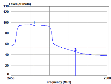
11g_TX_CH_11_Vertical-Avg
