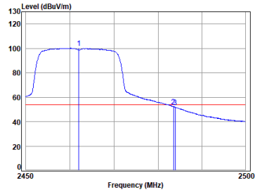
11n_HT(20M)_TX_CH_11_Horizontal-Avg
