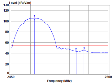
11b_TX_CH_11_Horizontal-Avg
