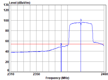
11n_HT(40M)_TX_CH_03_Horizontal-Avg
