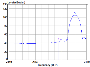
11b_TX_CH_01_Horizontal-Avg
