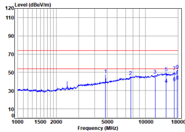
11b_TX_CH_06_Horizontal
