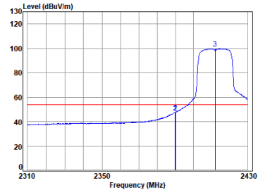
11n_HT(20M)_TX_CH_01_Horizontal-Avg
