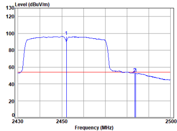
11n_HT(40M)_TX_CH_09_Horizontal-Avg
