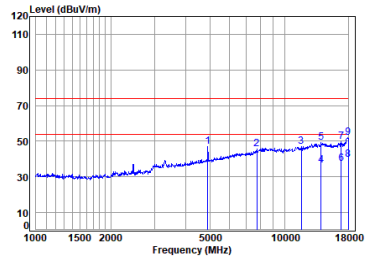
11b_TX_CH_11_Vertical
