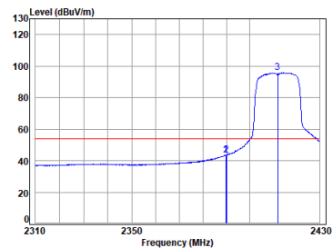
11n_HT(20M)_TX_CH_01_Vertical-Avg
