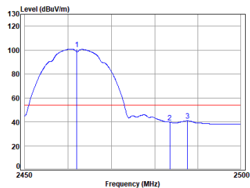
11b_TX_CH_11_Vertical-Avg
