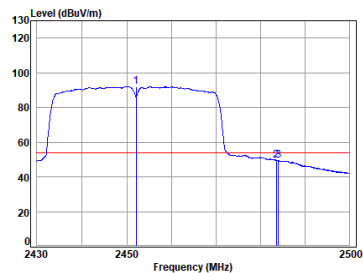
11n_HT(40M)_TX_CH_09_Vertical-Avg
