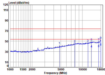
11n_20M_TX_CH_01_Vertical
