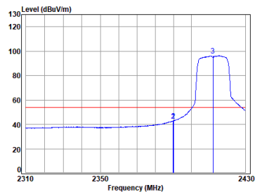
11g_TX_CH_01_Vertical-Avg
