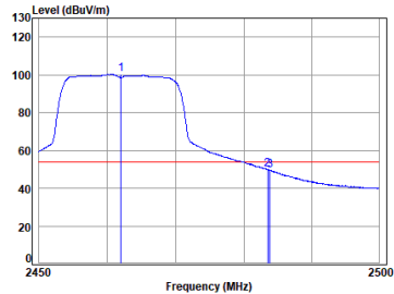
11g_TX_CH_11_Horizontal-Avg
