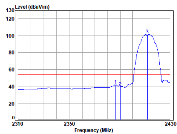
11b_TX_CH_01_Vertical-Avg
