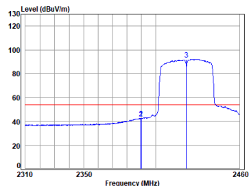
11n_HT(40M)_TX_CH_03_Vertical-Avg
