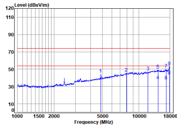
11n_20M_TX_CH_06_Vertical
