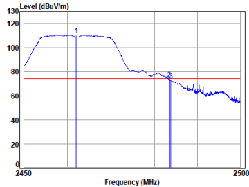
11n_HT(20M)_TX_CH_11_Horizontal-Peak
