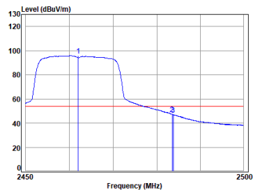
11n_HT(20M)_TX_CH_11_Vertical-Avg
