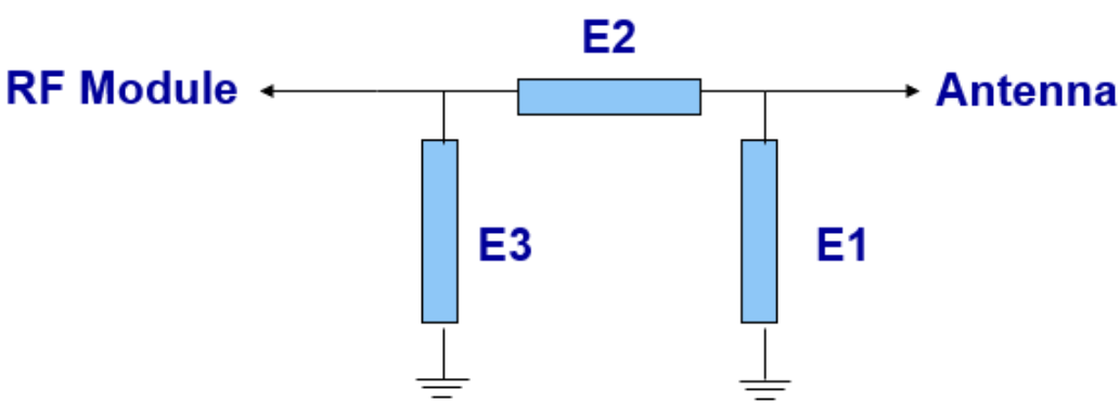
匹配电路
