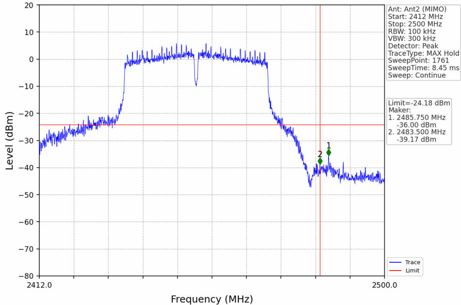
802.11n(HT40)_HCH_2452MHz_Ant2 (MIMO)_NTNV
