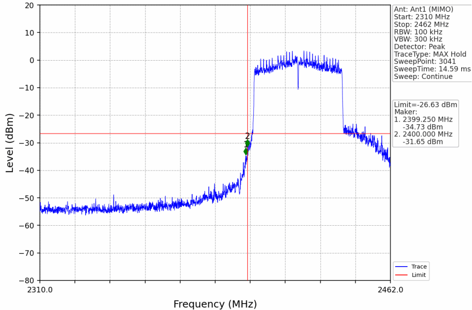
802.11ax(HEW40)_LCH_2422MHz_RU484_Left_Ant1 (MIMO)_NTNV
