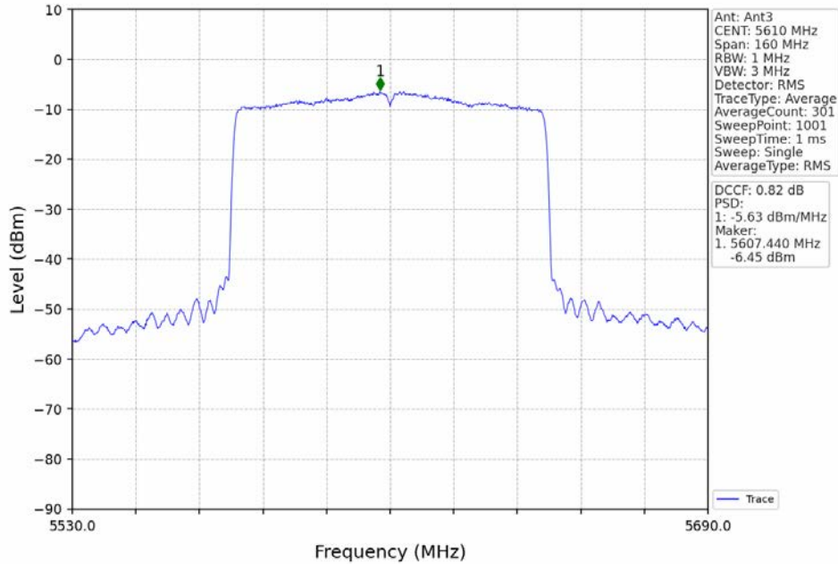
802.11ax(HEW80)_HCH_5610MHz_RU996_Left_MIMO_NTNV
