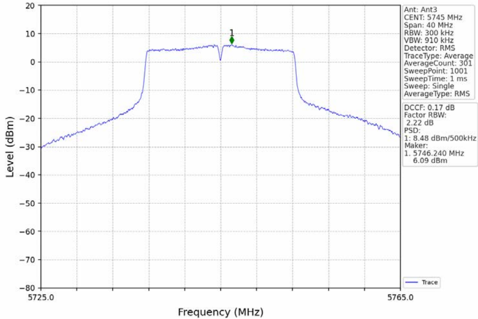
802.11a_LCH_5745MHz_MIMO_NTNV
