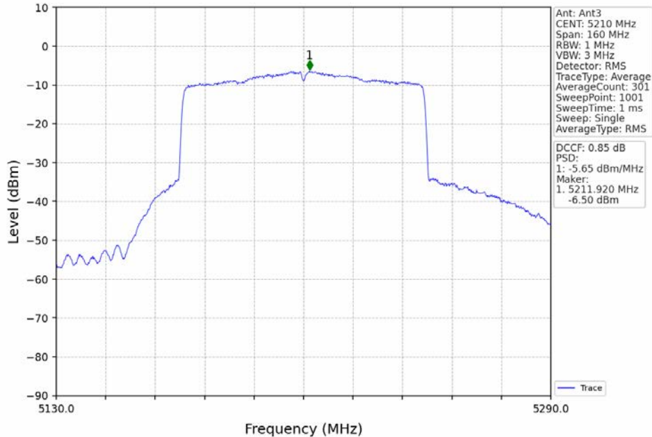
802.11ax(HEW80)_MCH_5210MHz_RU996_Left_MIMO_NTNV
