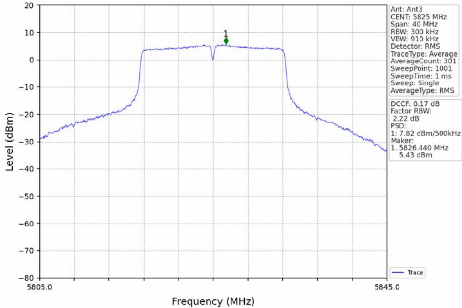
802.11a_HCH_5825MHz_MIMO_NTNV
