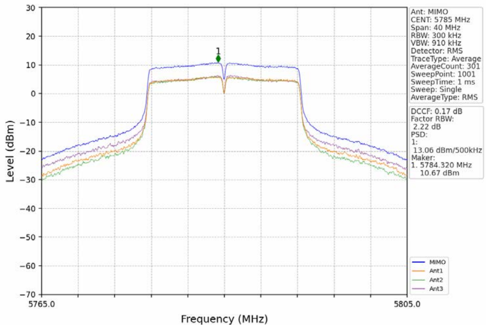
802.11a_MCH_5785MHz_MIMO_NTNV
