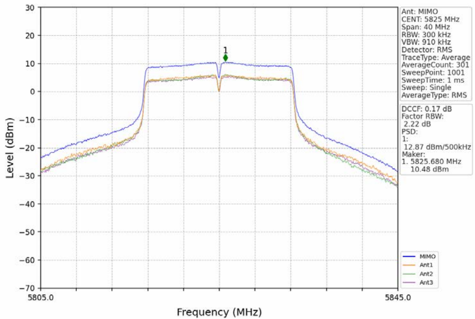
802.11a_HCH_5825MHz_MIMO_NTNV
