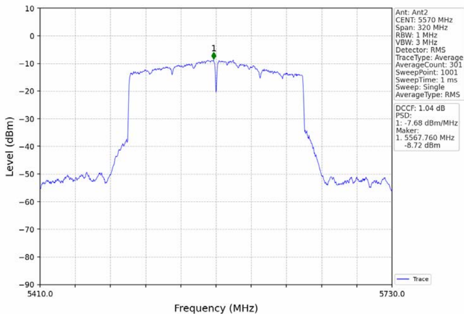
802.11ax(HEW160)_MCH_5570MHz_2xRU996_Left_Ant2_NTNV
