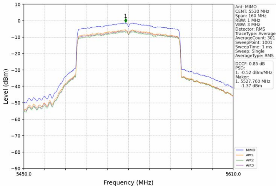
802.11ax(HEW80)_LCH_5530MHz_RU996_Left_MIMO_NTNV
