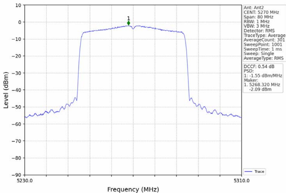
802.11ax(HEW40)_LCH_5270MHz_RU484_Left_Ant2_NTNV
