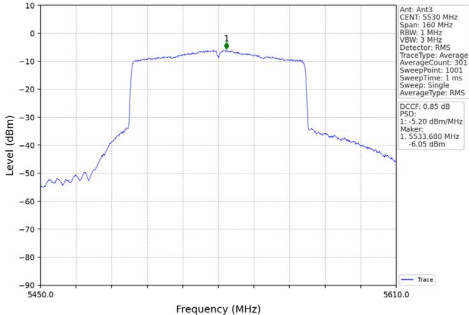
802.11ax(HEW80)_LCH_5530MHz_RU996_Left_MIMO_NTNV
