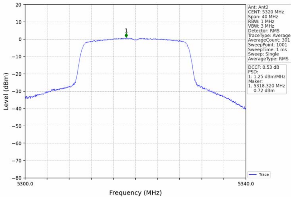
802.11ax(HEW20)_HCH_5320MHz_RU242_Left_Ant2_NTNV
