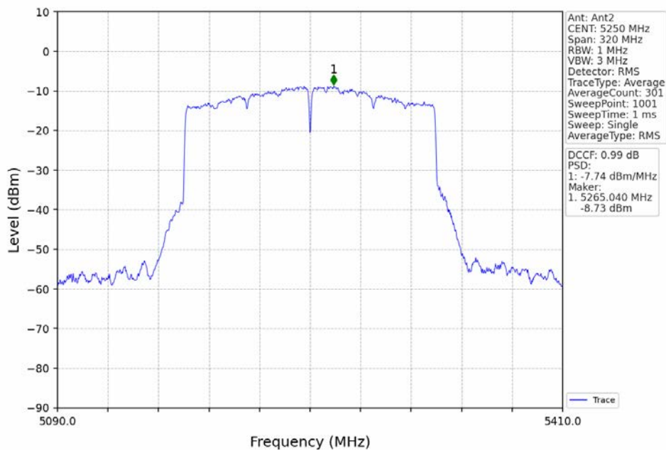
802.11ax(HEW160)_MCH_5250MHz_2xRU996_Left_Ant2_NTNV
