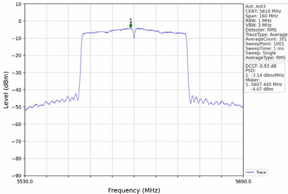
802.11ac(VHT80)_HCH_5610MHz_MIMO_NTNV
