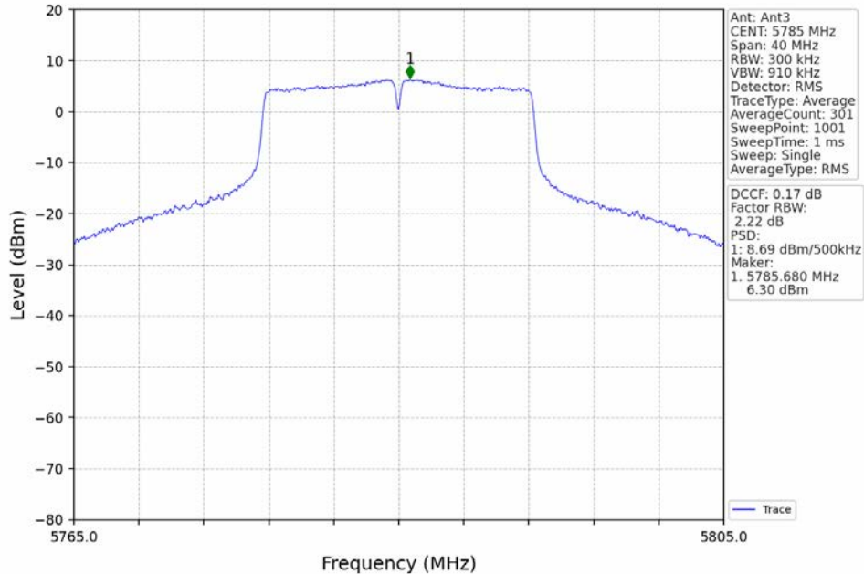
802.11a_MCH_5785MHz_MIMO_NTNV
