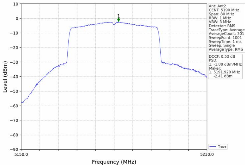
802.11ax(HEW40)_LCH_5190MHz_RU484_Left_Ant2_NTNV
