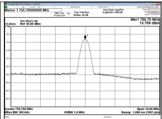
Upper 700MHz Band CW, DL
