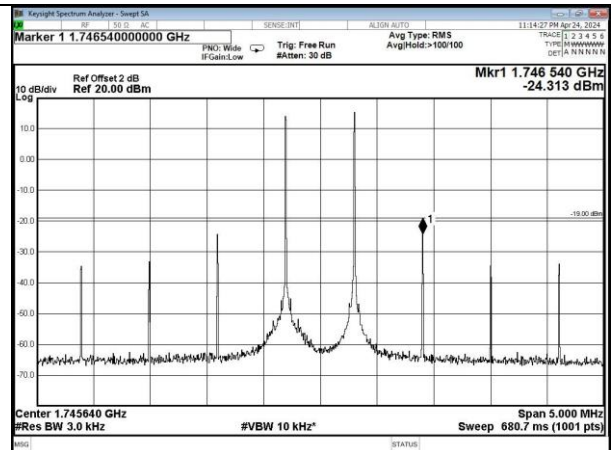
AWS Band AGC+10dB, UL
