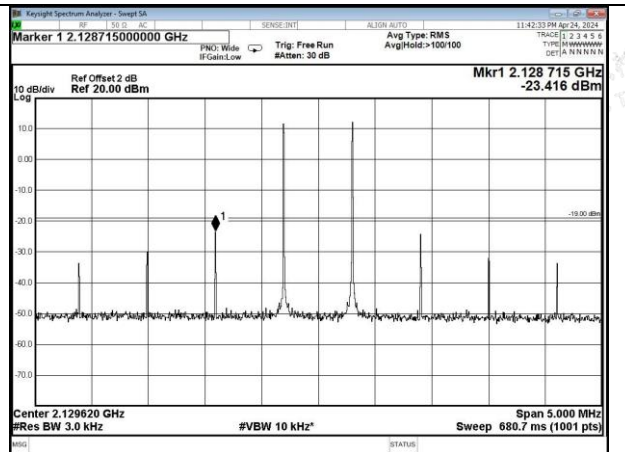
AWS Band AGC+10dB, DL
