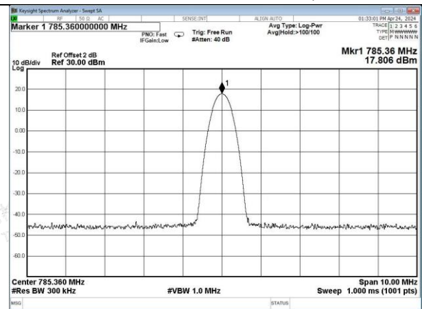
Upper 700MHz Band CW, UL
