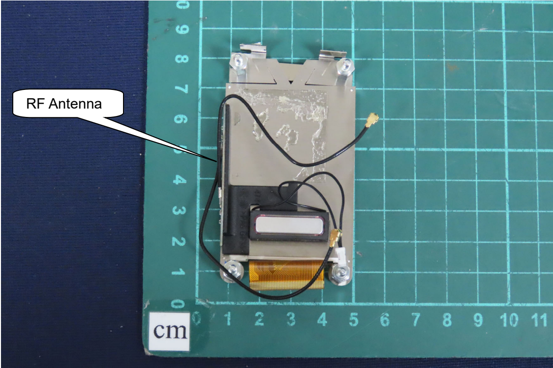
(19) EUT Photo
