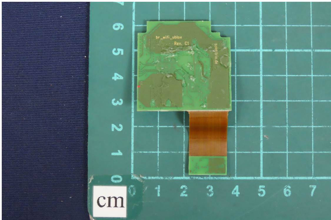
(18) EUT Photo
