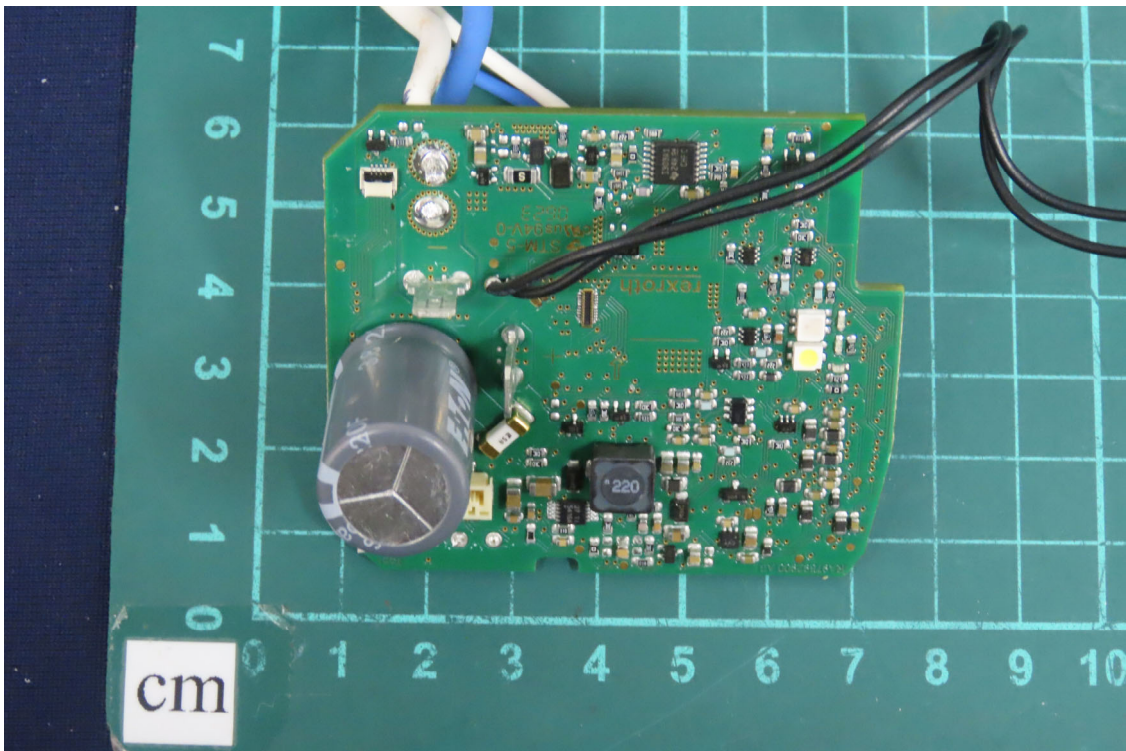
(30) EUT Photo
