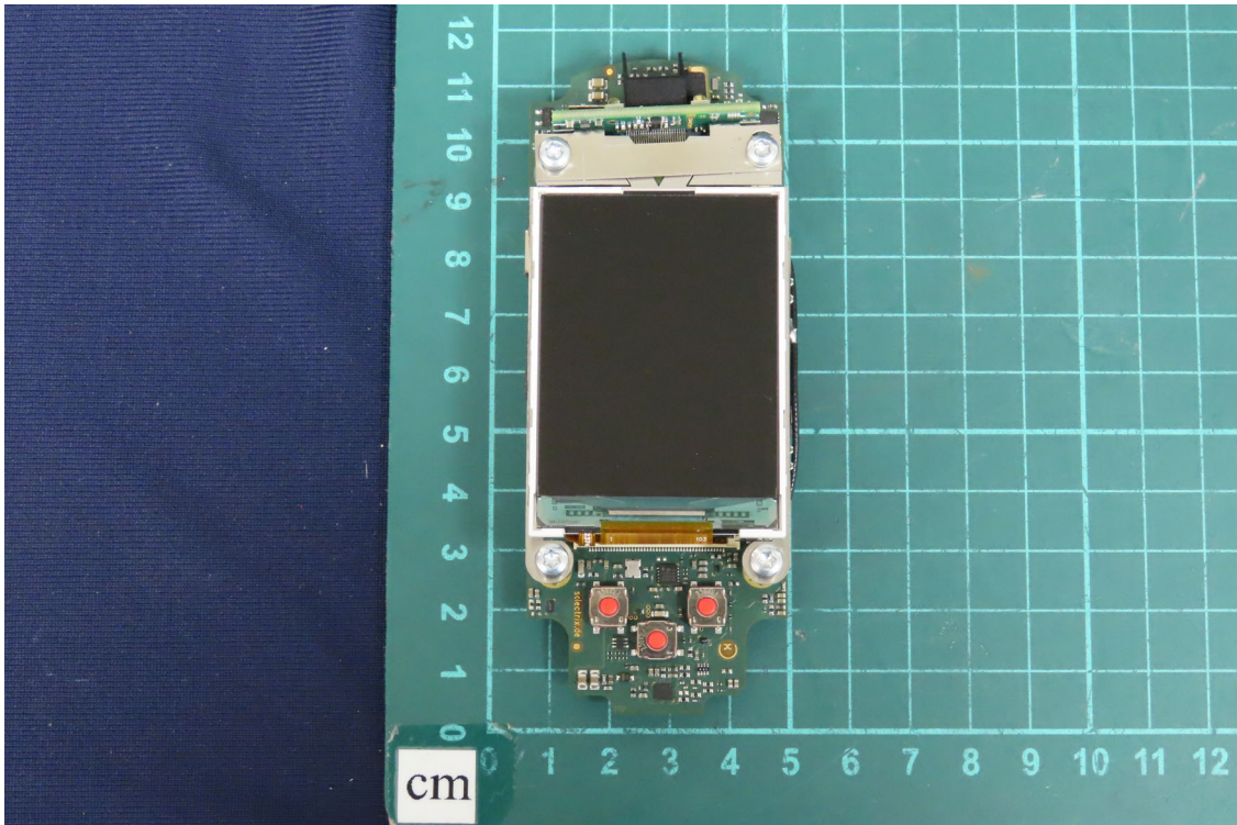
(40) EUT Photo
