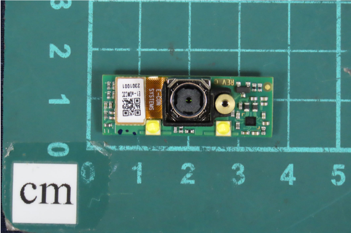
(44) EUT Photo
