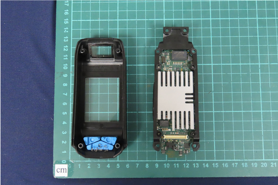
(36) EUT Photo
