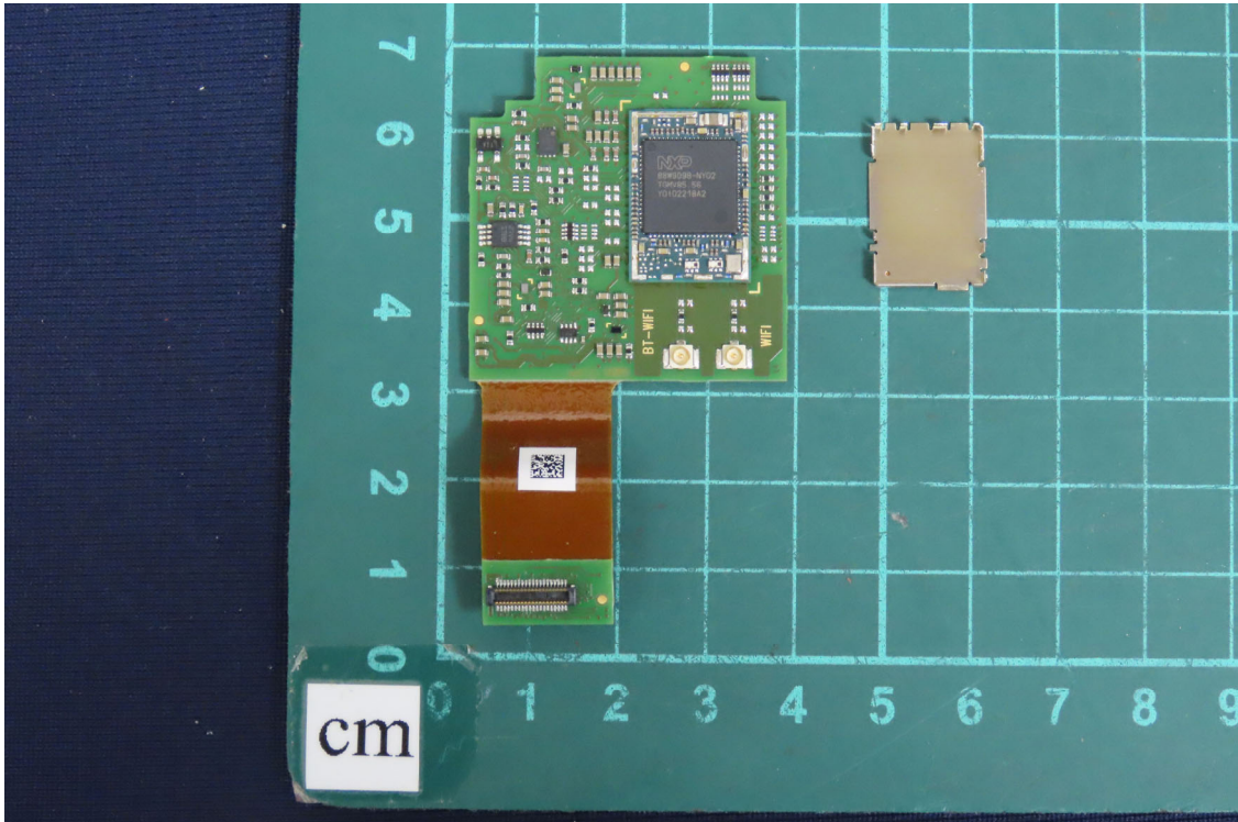
(47) EUT Photo
