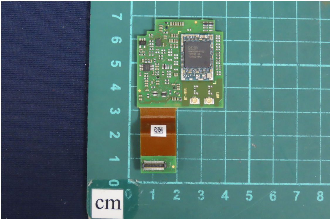
(48) EUT Photo
