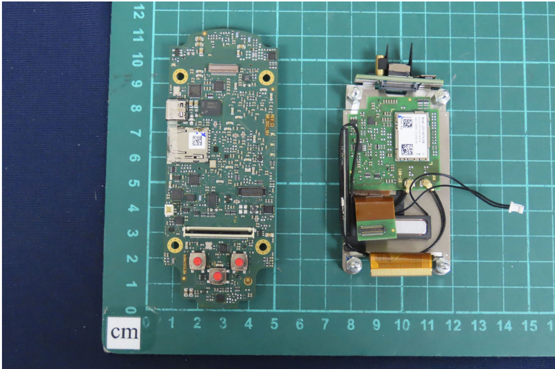
(41) EUT Photo
