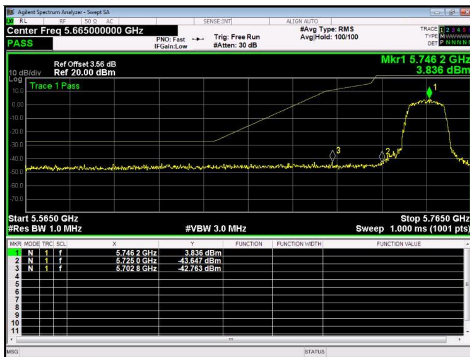
U-NII-3 802.11a right side
