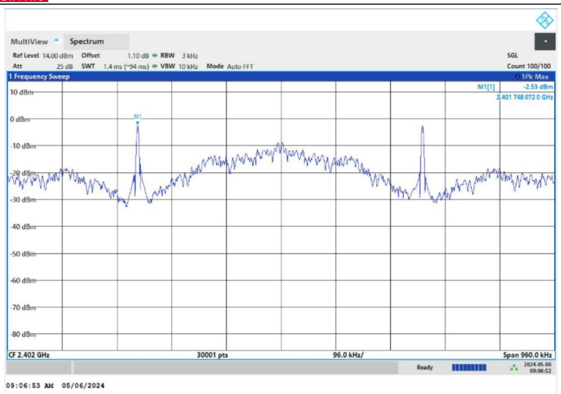
BLE_S8_Ant1_2402
