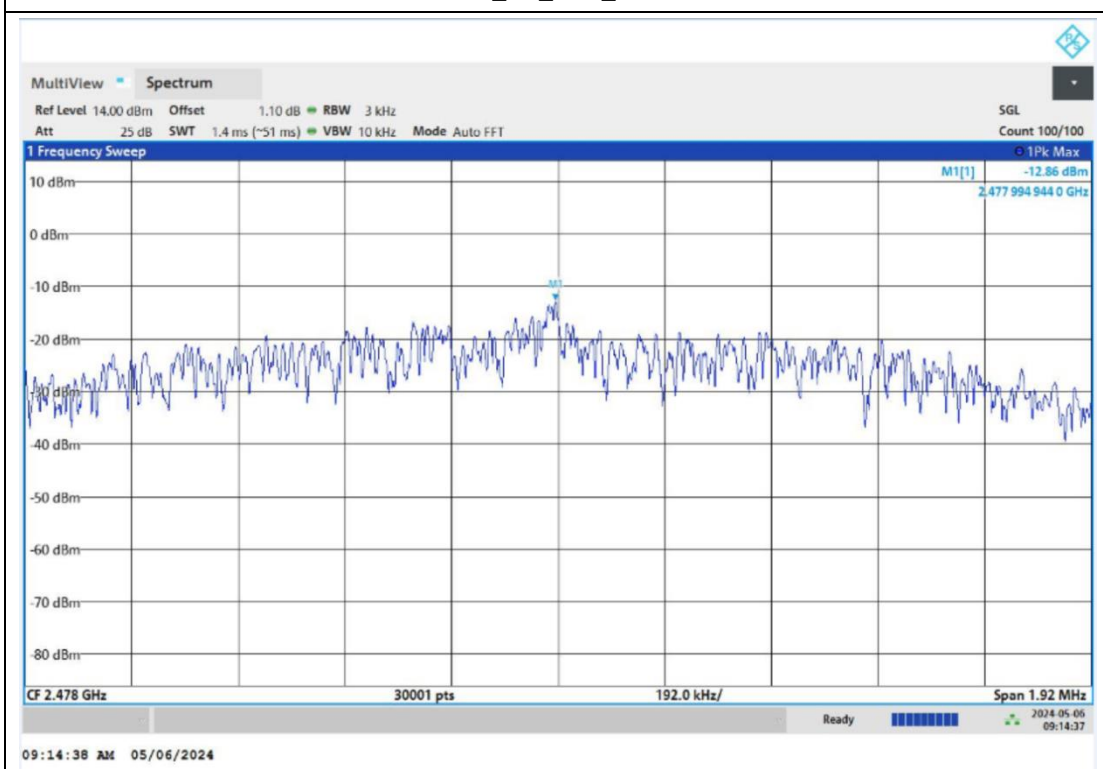
BLE_2M_Ant1_2478
