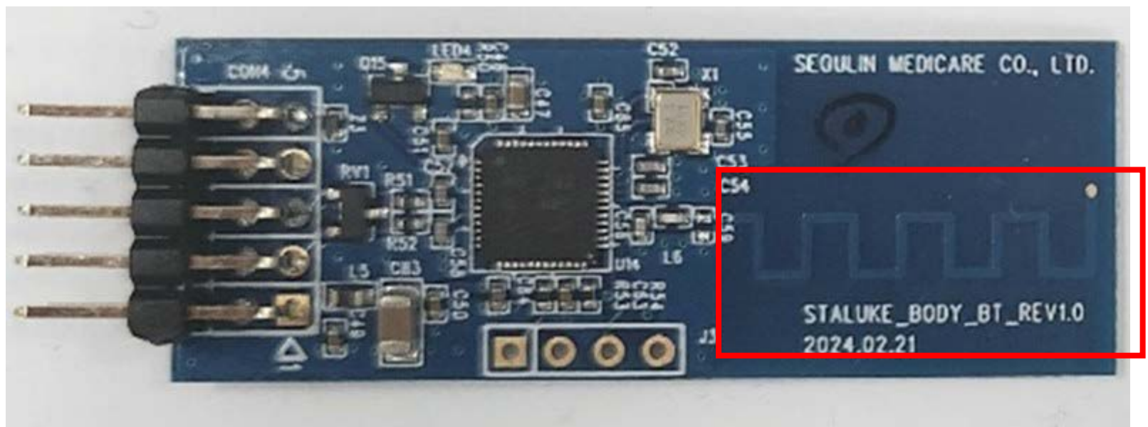
Body BLE Module Antenna Pattern & Value
