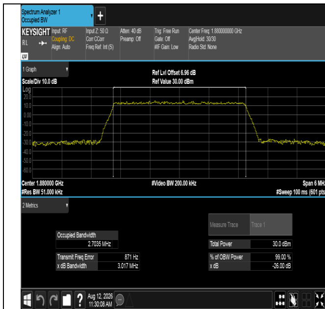
Band2-3MHz-QPSK-18900-15RB#0-PASS
