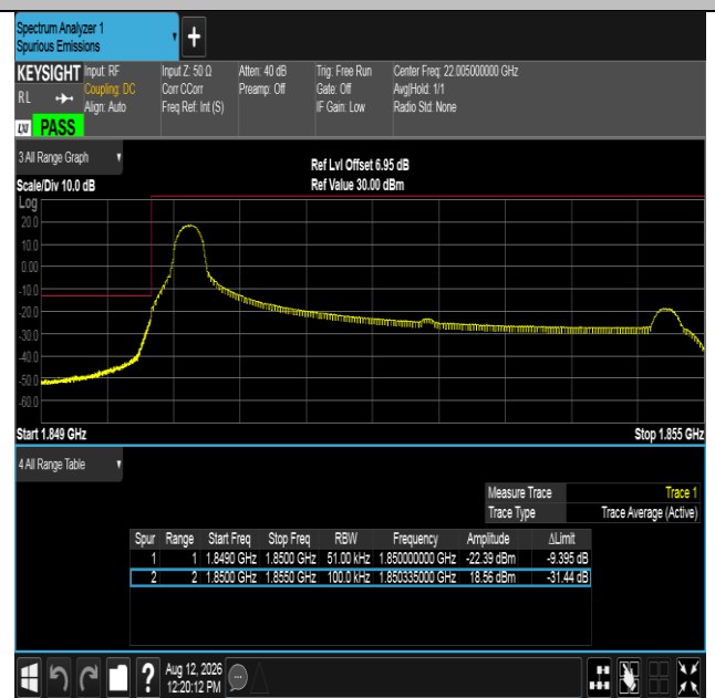
Band2-5MHz-16QAM-18625-1RB#0-PASS
