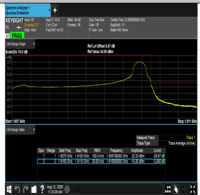
Band2-3MHz-QPSK-19185-1RB#14-PASS
