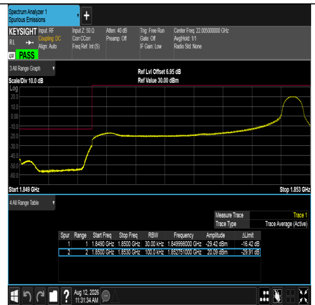
Band2-3MHz-QPSK-18615-1RB#14-PASS
