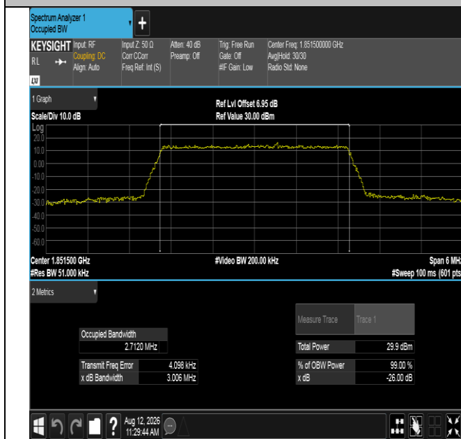
Band2-3MHz-QPSK-18615-15RB#0-PASS
