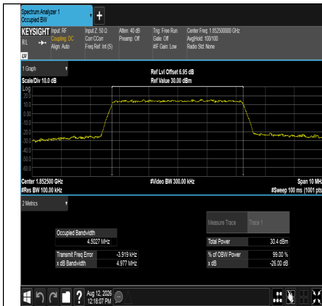
Band2-5MHz-QPSK-18625-25RB#0-PASS
