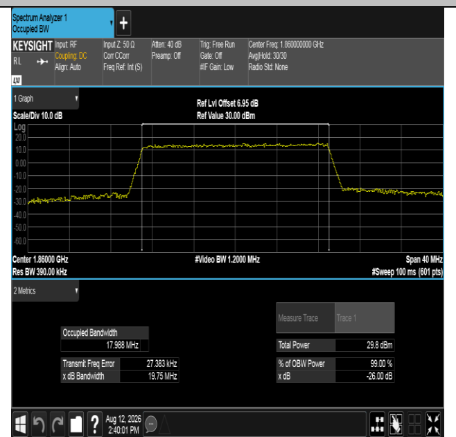
Band2-20MHz-16QAM-18700-100RB#0-PASS
