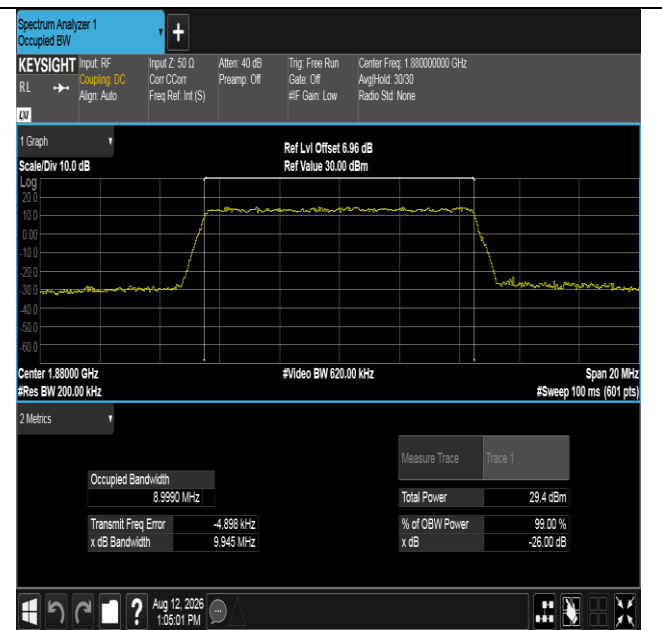
Band2-10MHz-16QAM-18900-50RB#0-PASS
