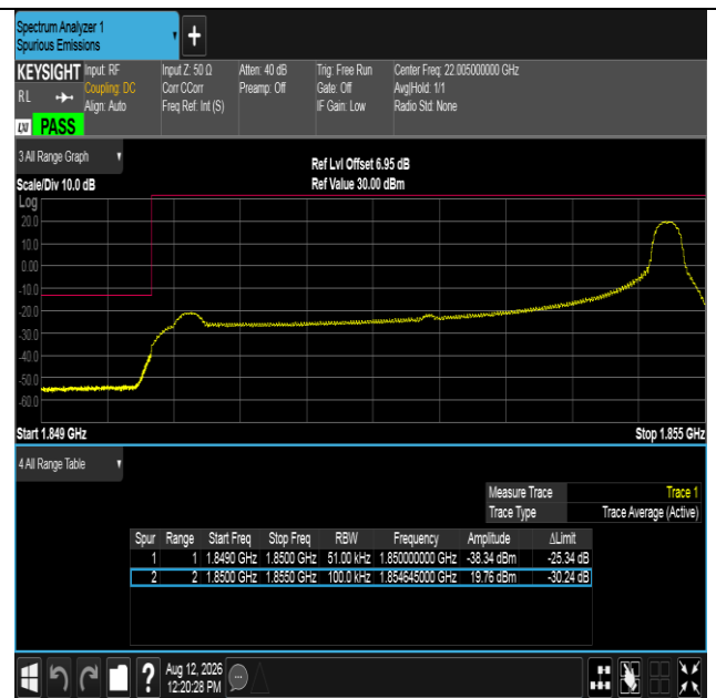
Band2-5MHz-QPSK-18625-1RB#24-PASS
