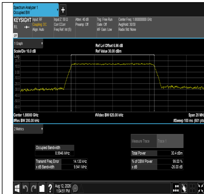
Band2-10MHz-QPSK-18900-50RB#0-PASS
