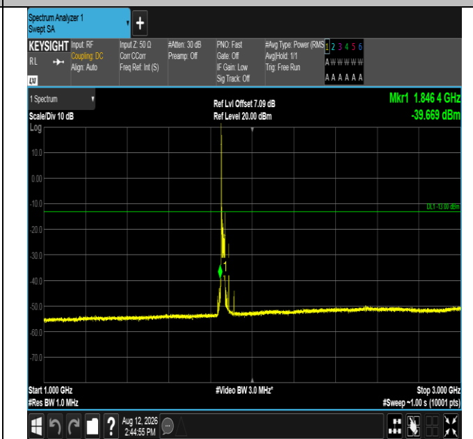
Band2-20MHz-QPSK-18700-1RB#0-1000~3000-PASS
