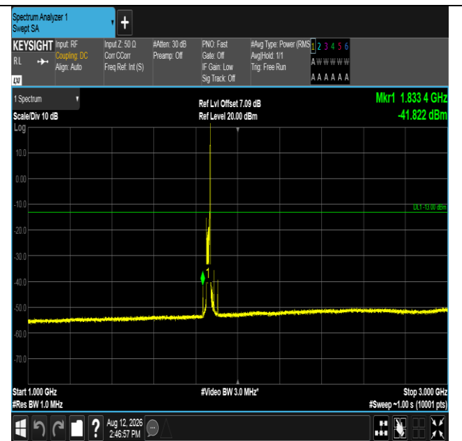
Band2-20MHz-QPSK-18700-1RB#99-1000~3000-PASS
