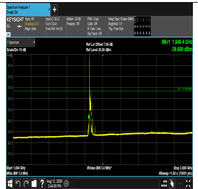
Band2-20MHz-QPSK-18700-1RB#0-1000~3000-PASS
