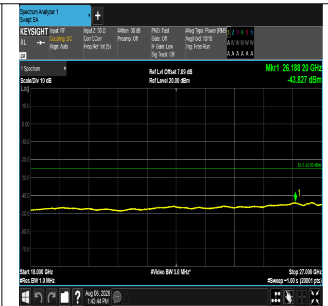
Band38-15MHz-QPSK-37825-1RB#0-18000~27000-PASS
