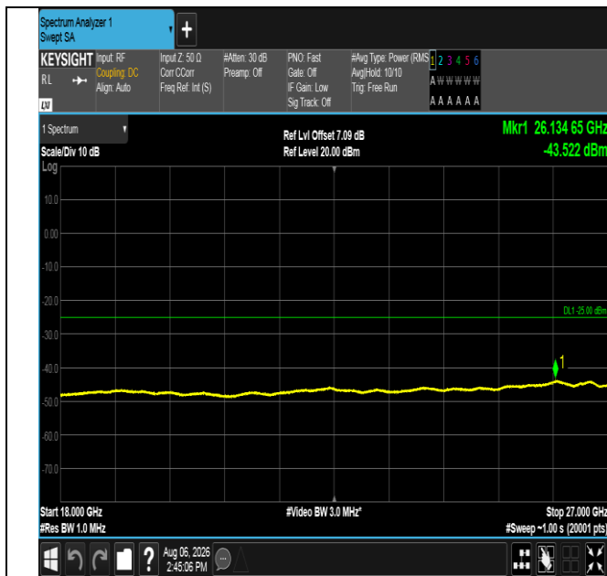
Band38-20MHz-QPSK-38000-1RB#99-18000~27000-PASS
