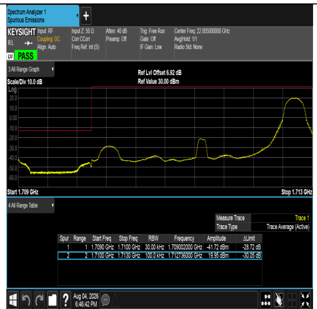
Band4-3MHz-QPSK-19965-1RB#14-PASS
