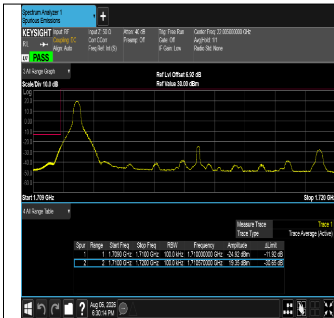
Band4-10MHz-QPSK-20000-1RB#0-PASS
