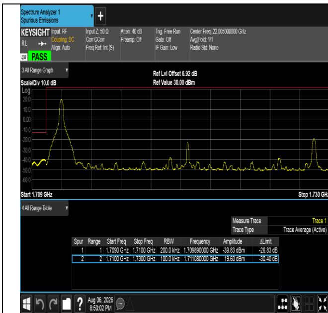
Band4-20MHz-QPSK-20050-1RB#0-PASS
