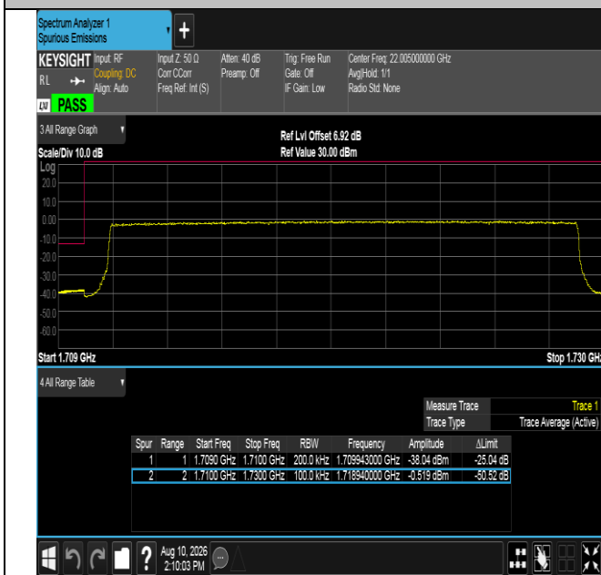
Band4-20MHz-QPSK-20050-100RB#0-PASS
