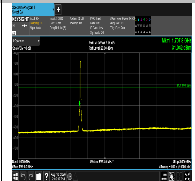
Band4-10MHz-QPSK-20000-50RB#0-1000~3000-PASS
