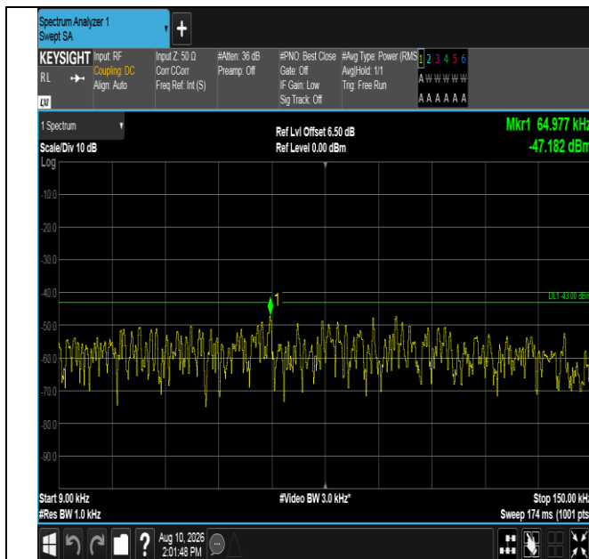
Band4-10MHz-QPSK-20000-50RB#0-0.009~0.15-PASS
