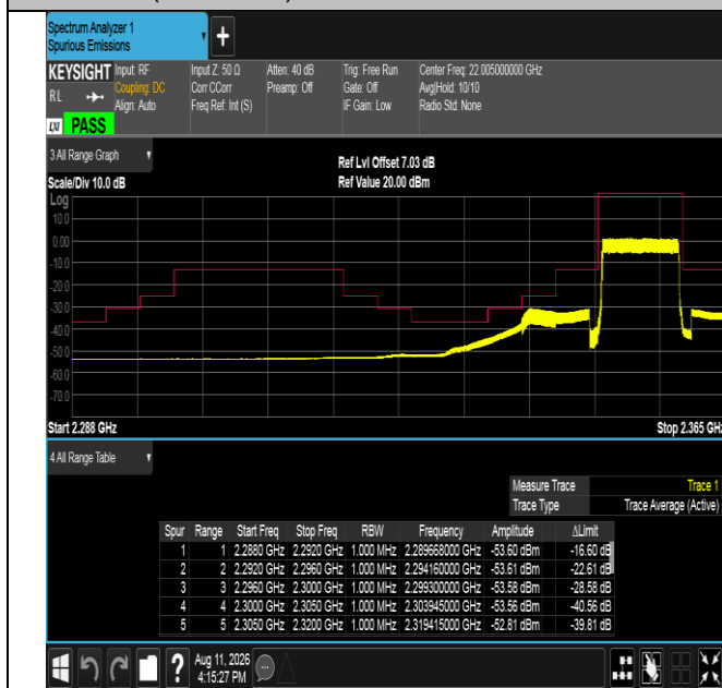
Band40(2350-2360)-10MHz-QPSK-39200-50RB#0-PASS
