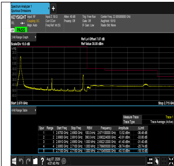
Band41-20MHz-QPSK-41490-1RB#0-PASS
