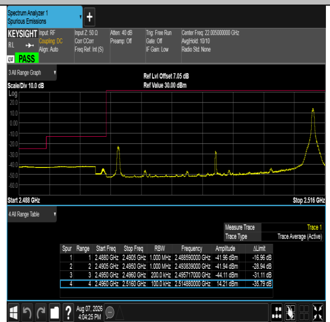
Band41-20MHz-QPSK-39750-1RB#99-PASS
