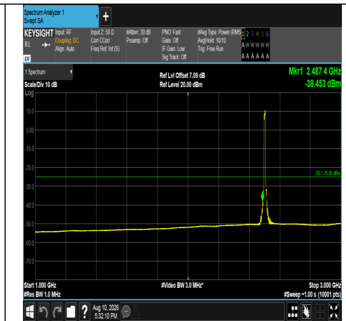
Band41-10MHz-QPSK-39700-50RB#0-1000~3000-PASS
