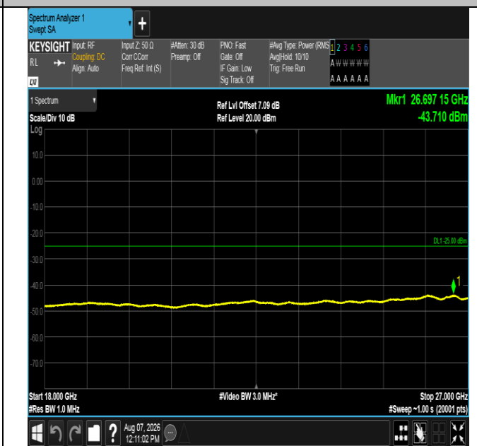
Band41-5MHz-QPSK-40620-25RB#0-18000~27000-PASS
