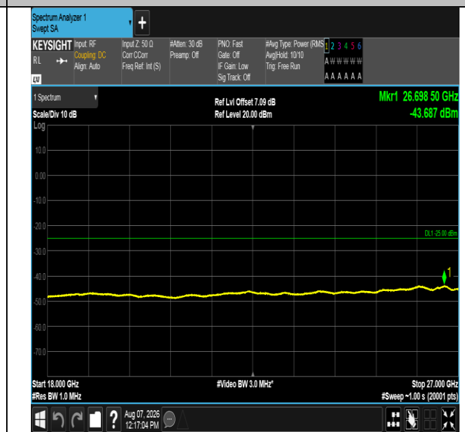
Band41-5MHz-16QAM-41565-1RB#0-18000~27000-PASS
