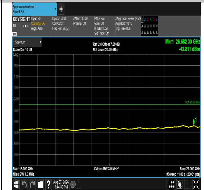
Band41-15MHz-16QAM-41515-1RB#0-18000~27000-PASS
