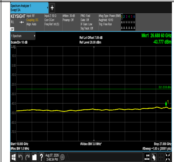
Band41-15MHz-16QAM-41515-1RB#74-18000~27000-PASS
