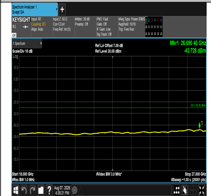
Band41-20MHz-QPSK-41490-1RB#99-18000~27000-PASS
