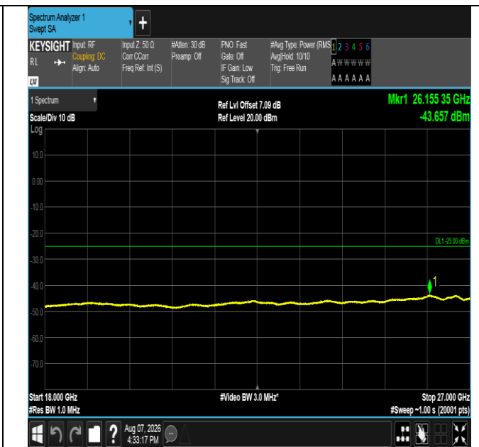
Band41-20MHz-16QAM-41490-1RB#0-18000~27000-PASS
