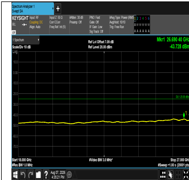
Band41-20MHz-QPSK-41490-1RB#99-18000~27000-PASS
