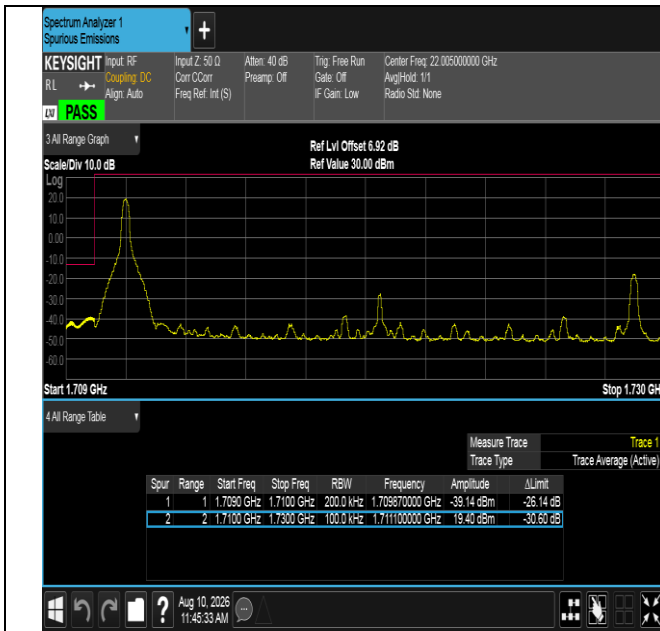
Band66-20MHz-QPSK-132072-1RB#0-PASS
