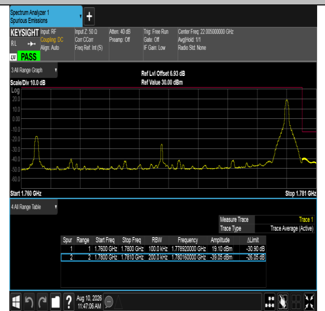
Band66-20MHz-QPSK-132572-1RB#99-PASS
