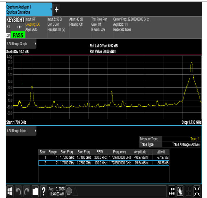
Band66-20MHz-QPSK-132072-1RB#99-PASS
