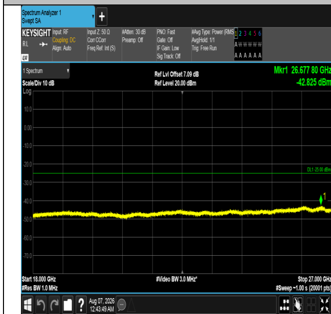
Band7-20MHz-QPSK-20850-1RB#99-18000~27000-PASS
