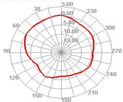
5050.000MHz E1
