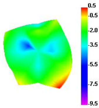
2500.000MHz E1
