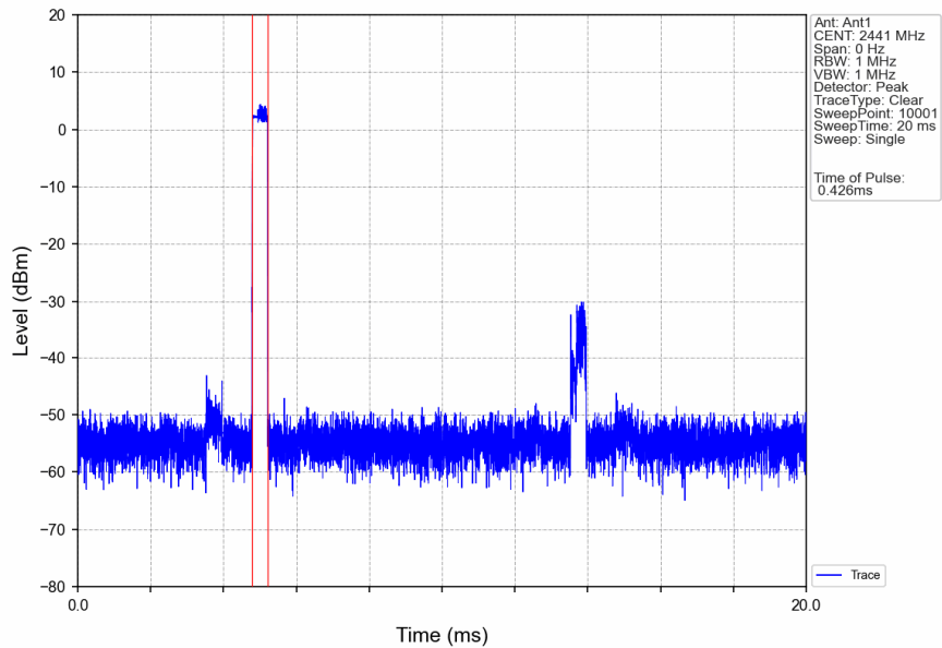
8DPSK_3DH1_HOPP_Ant1_NTNV
