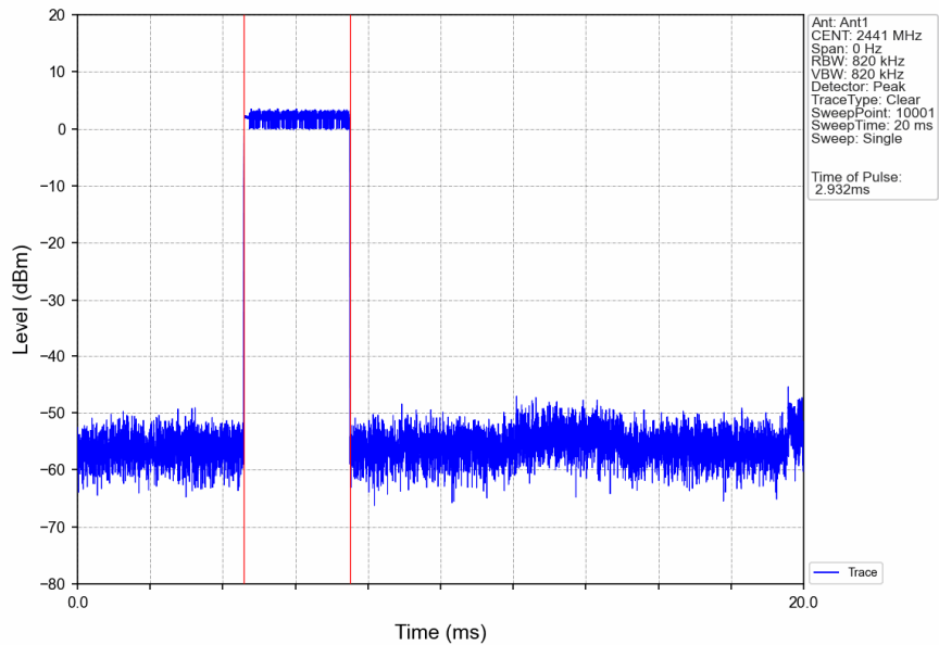
Pi/4DQPSK_2DH5_HOPP_Ant1_NTNV
