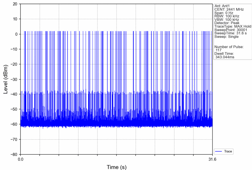
Pi/4DQPSK_2DH5_HOPP_Ant1_NTNV
