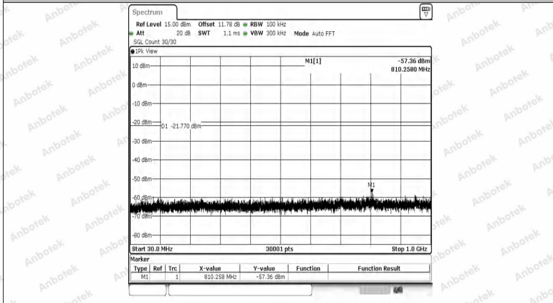
2.4G-Ant1-2441-30~1000-PASS
