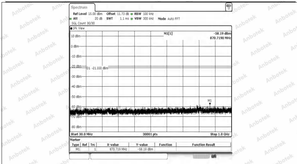
2.4G-Ant1-2480-30~1000-PASS
