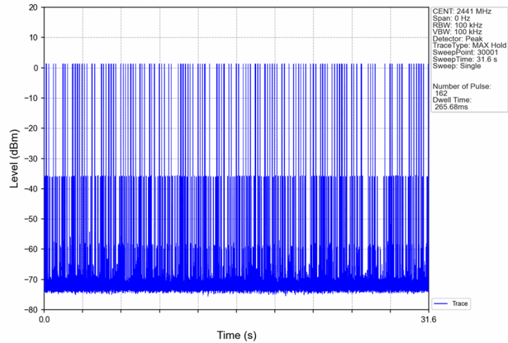
Pi/4DQPSK_2DH3_HOPP_Ant1_NTNV
