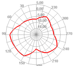
5500.000MHz E2
