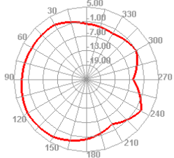
5500.000MHz H
