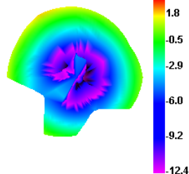
5150.000MHz E1
