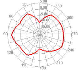
5850.000MHz E2
