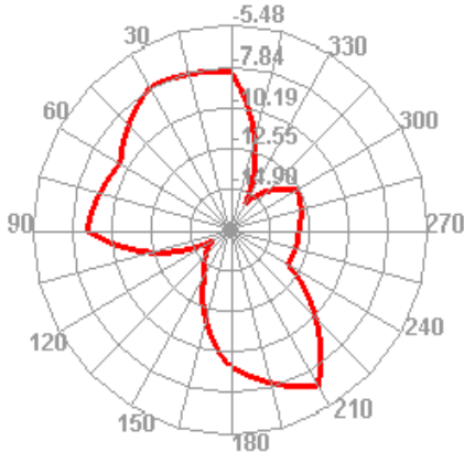
2400.000MHz E1
