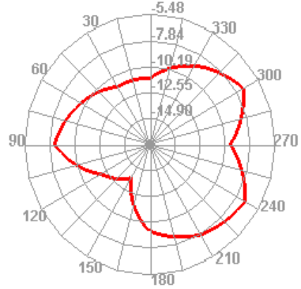
2400.000MHz E2
