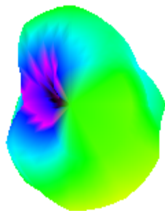
2400.000MHz
