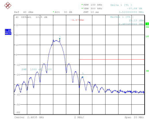
Right Side-2480MHz
