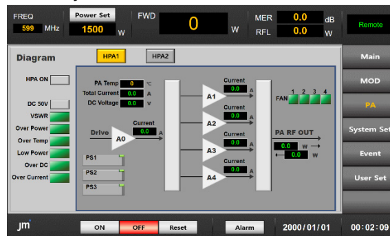
HPA1
