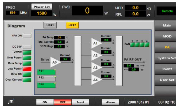
HPA2
