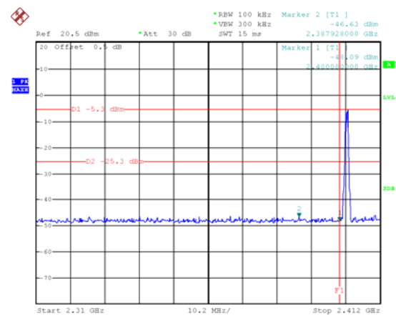
BLE (1M): Band edge-left side
