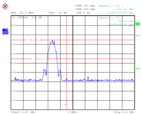
BLE (2M): Band edge-right side
