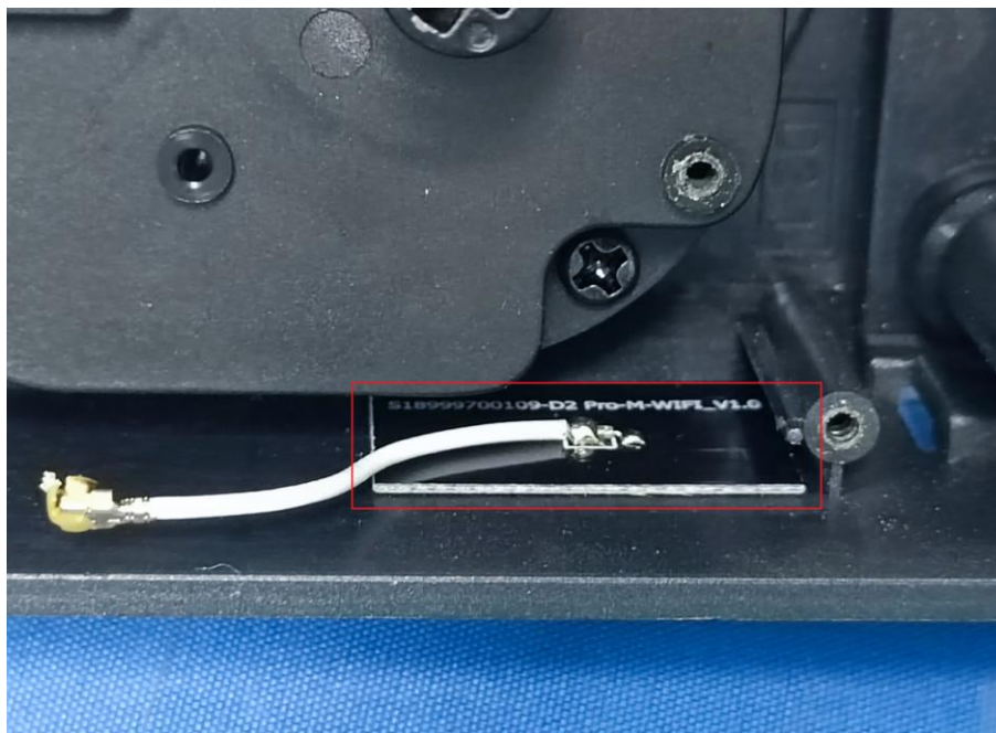
2.4G WiFi ANT & BLE ANT0
