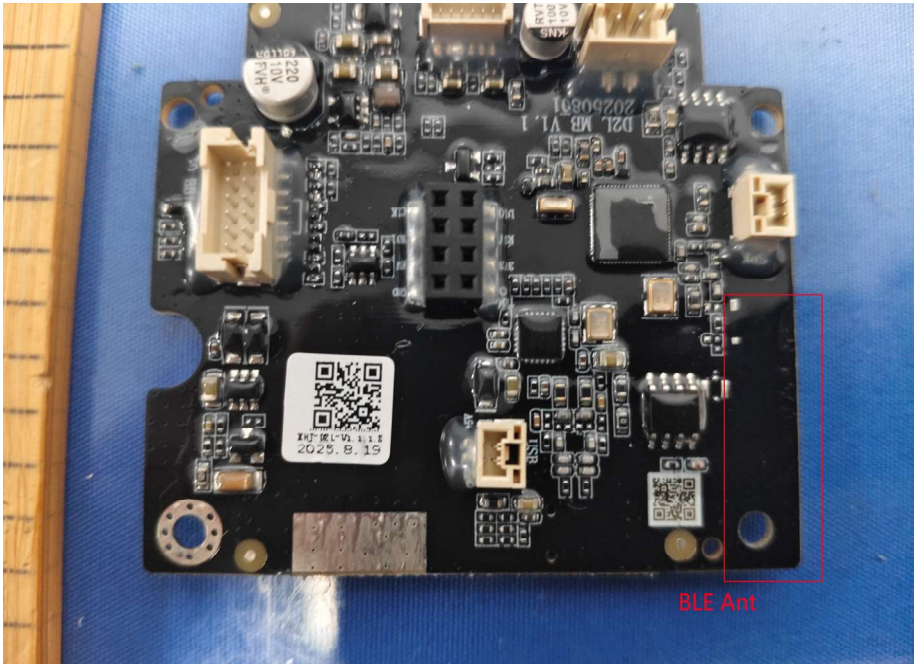
BLE Antenna
