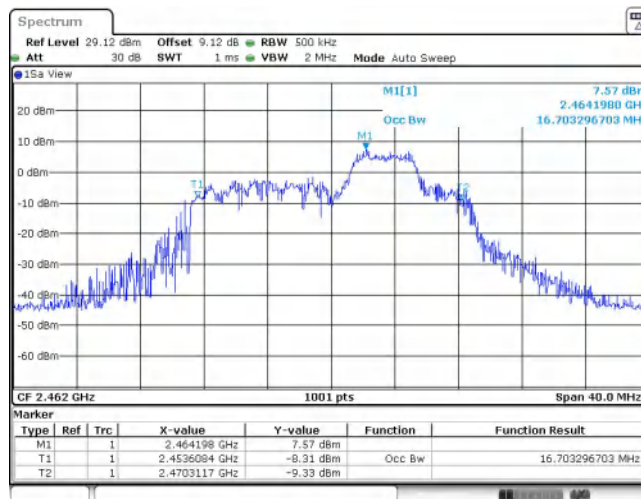
11AX20SISO_Ant1_2462_52Tone_RU37
