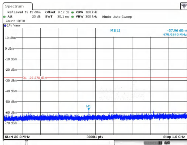
11AX40SISO_Ant1_2452_30~1000
