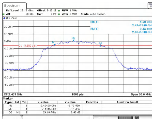
11AX40SISO_Ant1_2437
