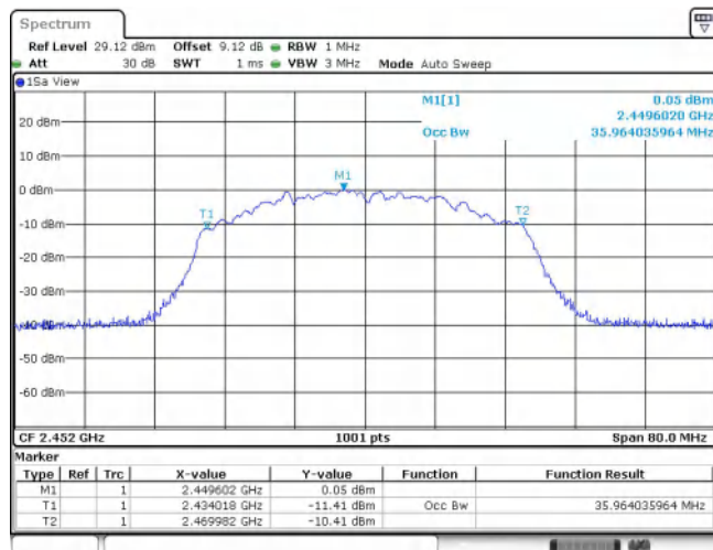
11AX40SISO_Ant1_2452
