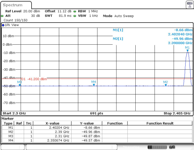
BLE_1M_Ant1_Low_2402_AV
