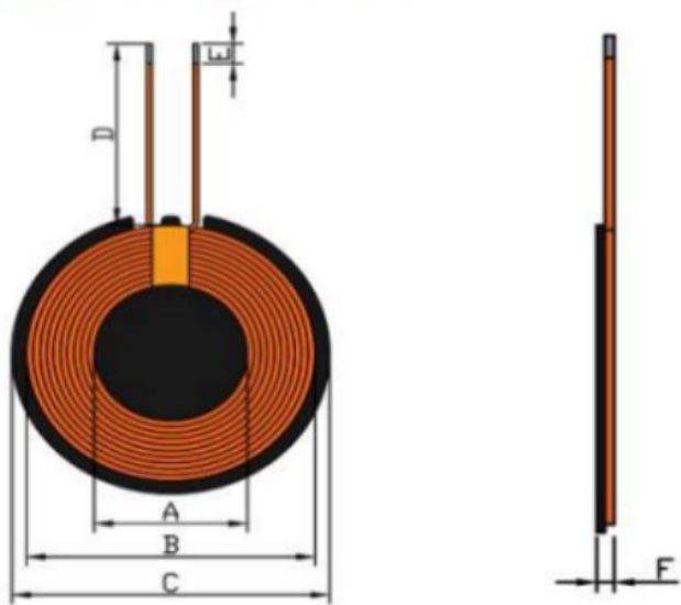
产品尺寸说明 Product Size(单位: MM)
