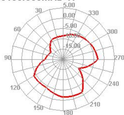
5150.000MHz H
