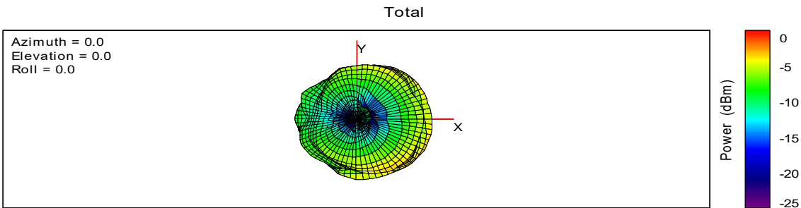
2440MHz TRP 1
