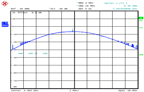
Low -6.48dBm
