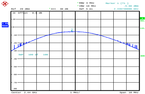
Middle -5.66dBm
